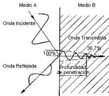
Fig. 2: Reflexión, absorción y transmisión de una onda al pasar, de un medio, a otro electromagnéticamente distinto
