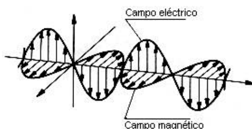
Fig. 1: Representación de una onda electromagnética
